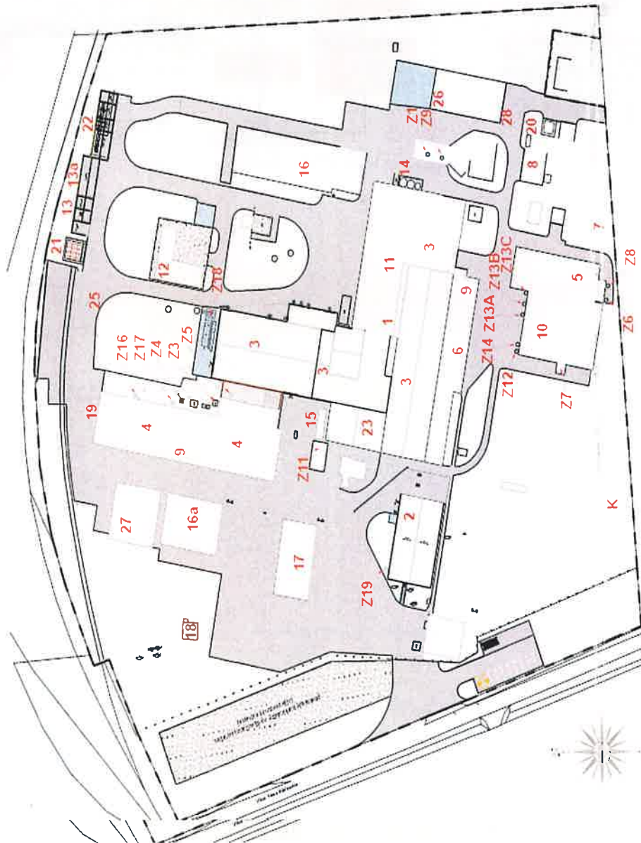
Prilog 1: Situacija postrojenja sa naznačenim tehnološkim cjelinama i mjestima emisija
